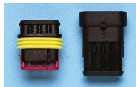
4 kontaktu Ligzda Art.Nr. 0555 103 4 Spraudnis 0555 102 4
