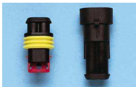
2 kontaktu Ligzda Art.Nr. 0555 103 2 Spraudnis 0555 102 2
