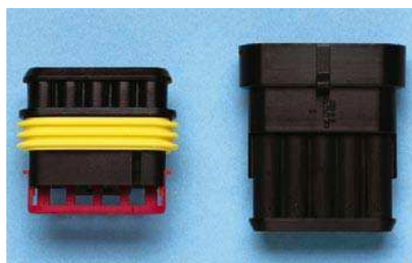
5 kontaktu Ligzda Art.Nr. 0555 103 5 Spraudnis 0555 102 5
